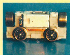
Antrieb mit drei veränderlichen Achsständen und 2 Schwungmassen
